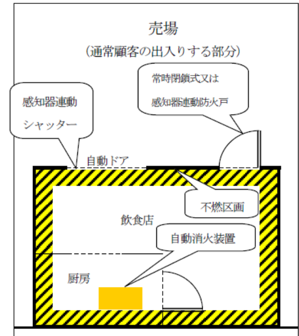
例4 飲食店が売場に面している場合 (煮沸行為をする厨房)
