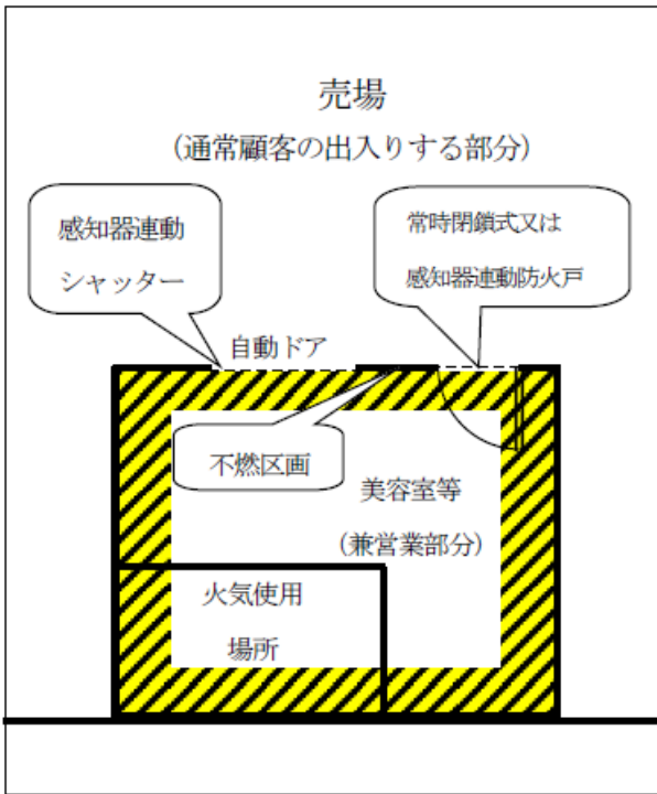
例1 美容室等が不燃区画されている場合
