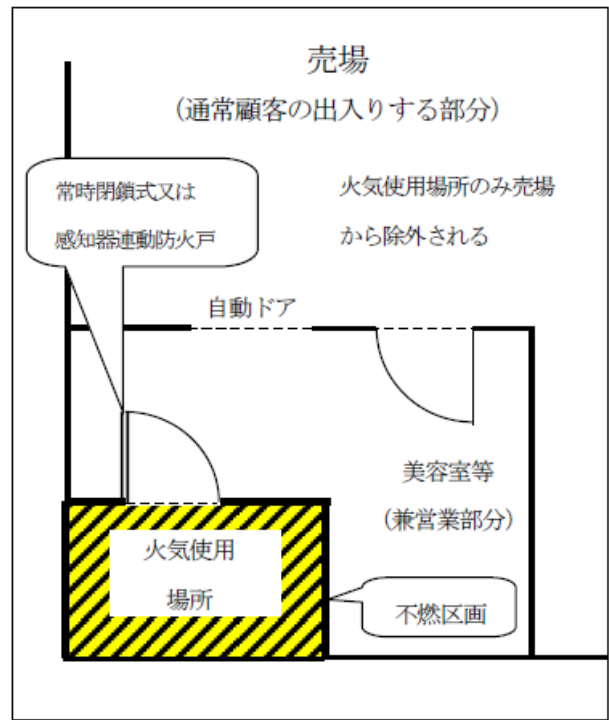
例2 美容室等の火気使用場所が不燃区画されている場合
