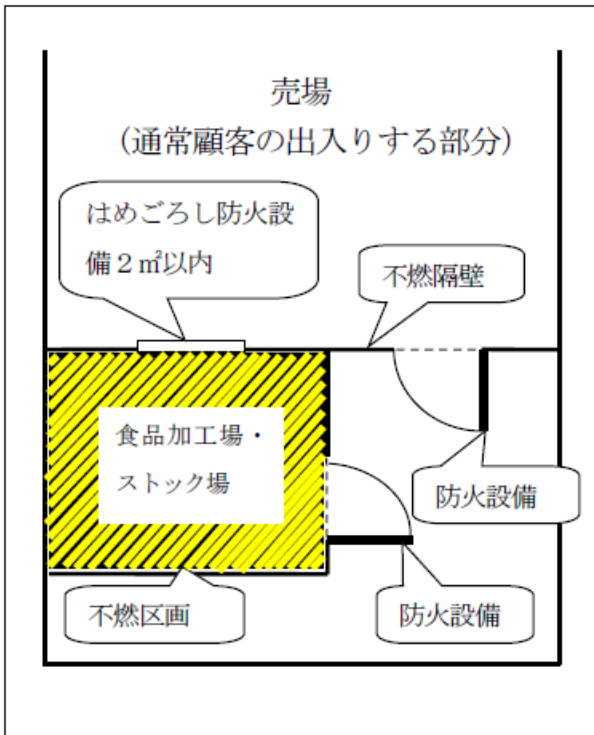
例3 バックヤード等及び加工場等開口部
