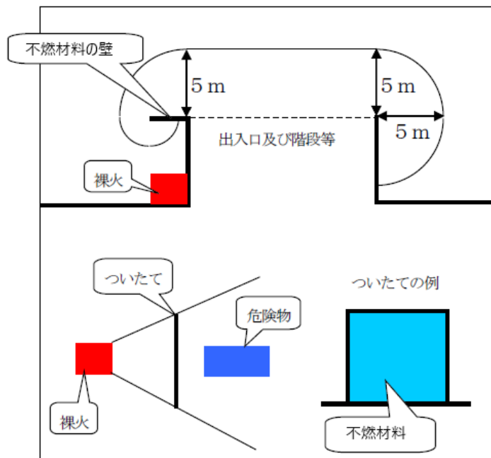
不燃材料の壁で防火上有効に遮断した場合の例 （避難口・階段等からの距離）
