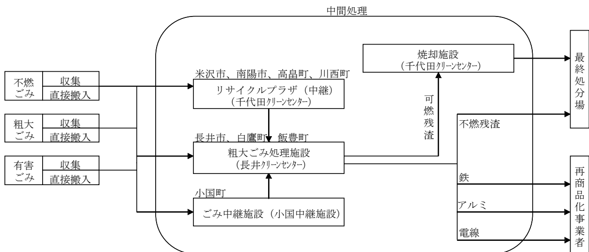
[図4] 不燃ごみ及び粗大ごみ処理体系
